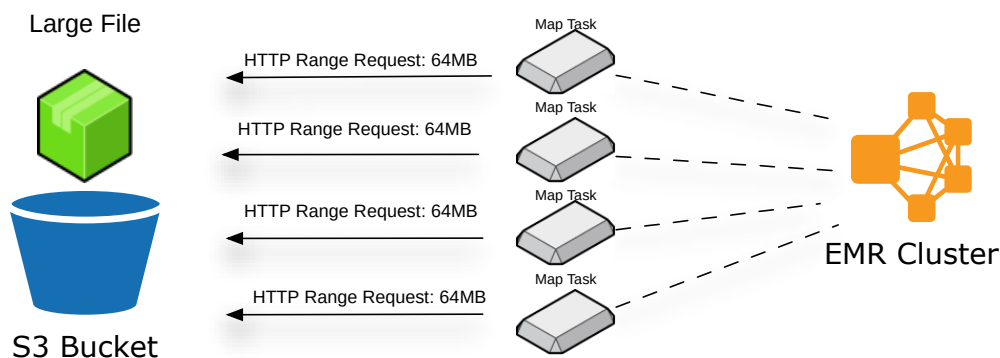
図 8: Amazon EMR の HTTP レンジリクエストの使用
